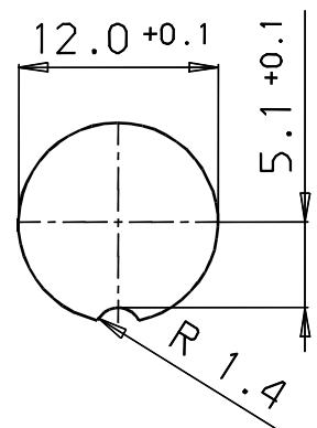
Montageausschnitt M 2:1
